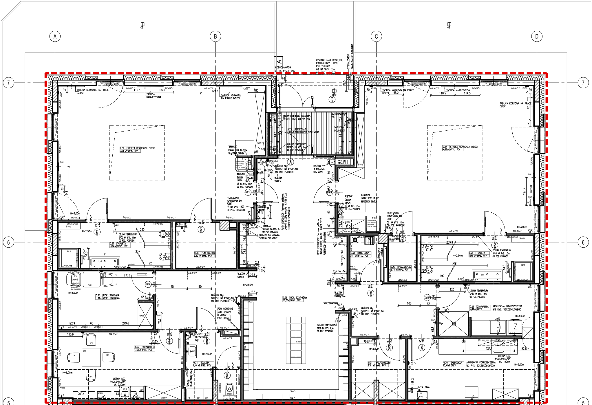
RZUT STREFY REKREACJI DZIECI skala 1:100
